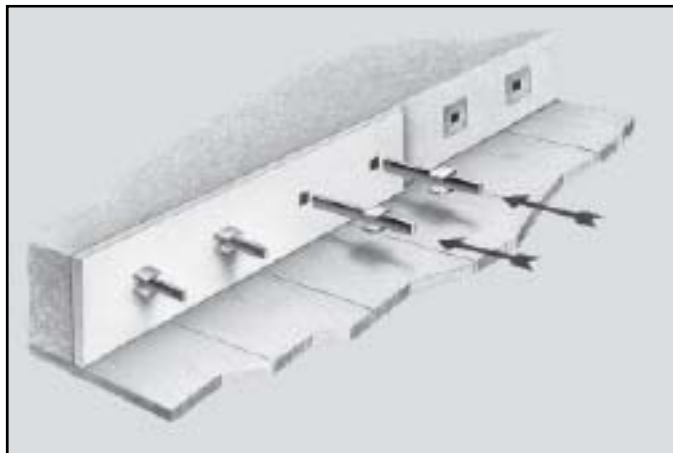
Na het ontkisten van de eerste stort voegenvulmateriaal plaatsen en de Cret®-deugel in de huls plaatsen
