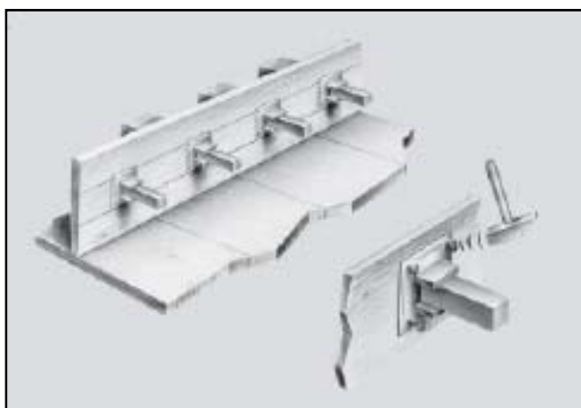
De Cret®-huls waterpas op de bekisting spijkers
